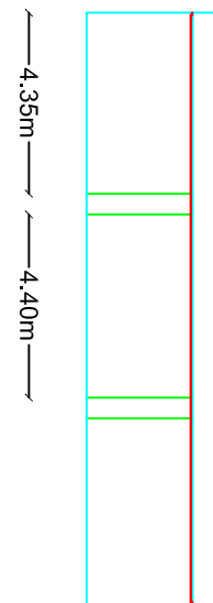
SECCION 4-4
